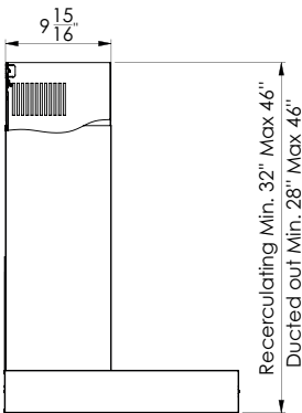
Partie latérale de la hotte
