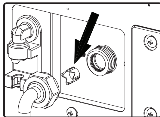
Emplacement du clapet antiretour de la pompe de vidange
