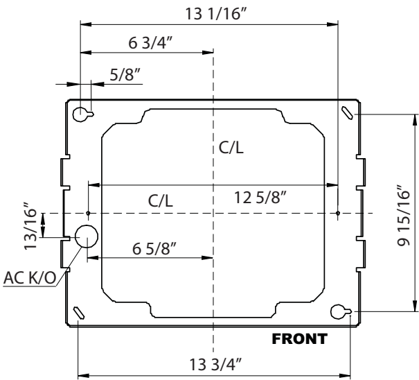
CADRE DE FIXATION SUPÉRIEUR (vue du dessus)
